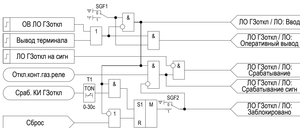
Рисунок 2.17 – Функциональная схема «ЛО ГЗоткл»
