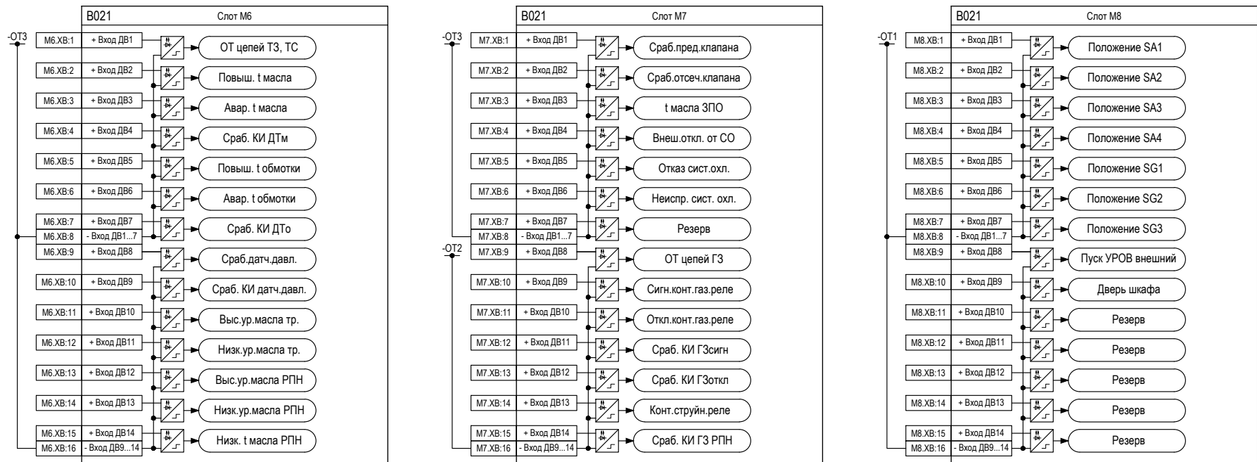
Рисунок Ж.3 – Подключение дискретных входов и выходов к внутренним сигналам алгоритмов для плат в слотах M6-M8
