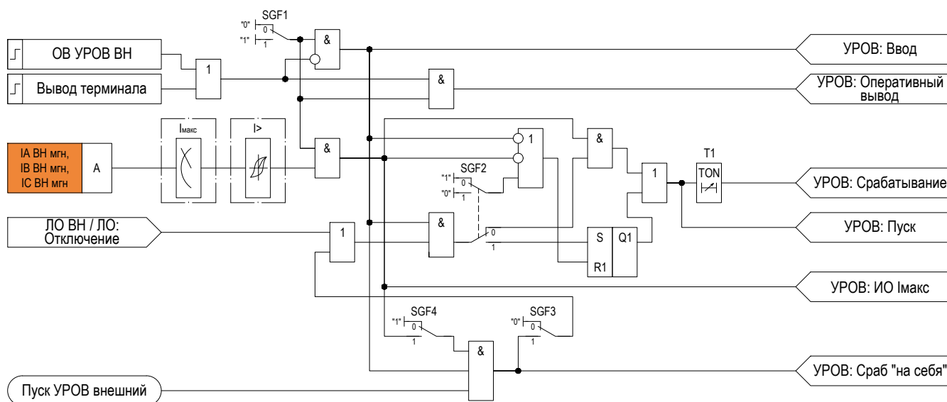
Рисунок 2.31 – Функциональная схема «УРОВ»
