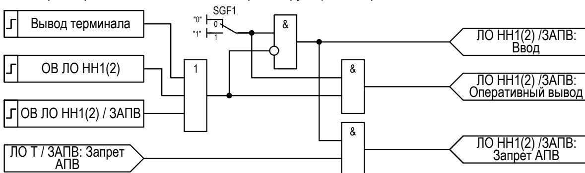
Рисунок 2.30 – Функциональная схема «Запрет АПВ»
